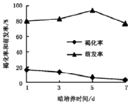
图1 不同时间的暗培养对腋芽褐化的影响
